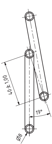
B-B ( 1 : 1 )
