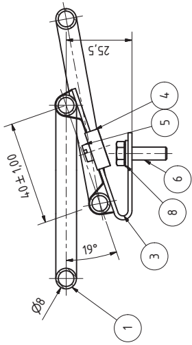
A-A ( 1 : 1 )
